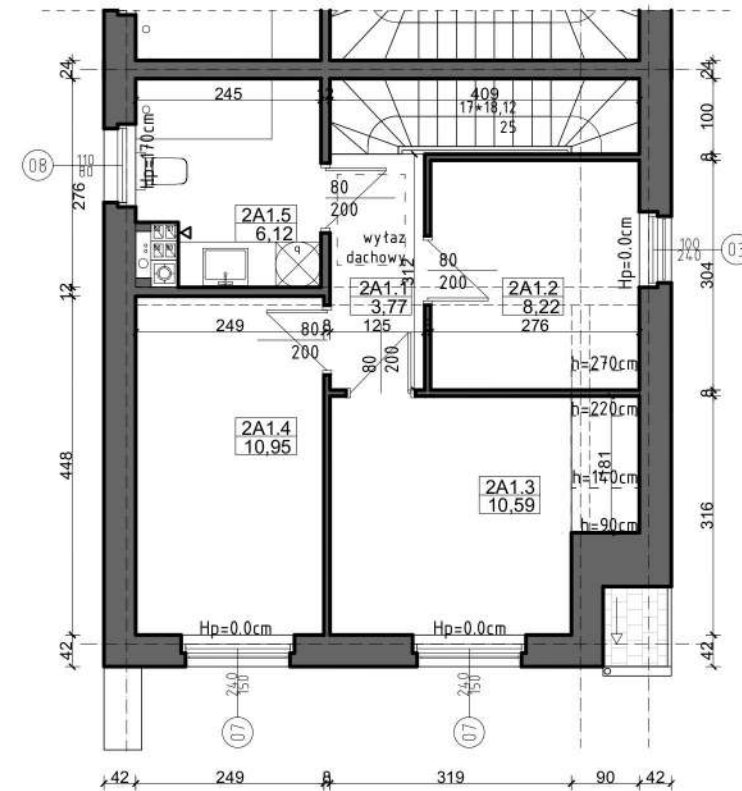
RZUT PODDASZA
