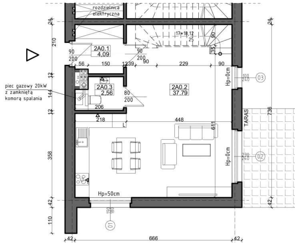
RZUT PARTERU
